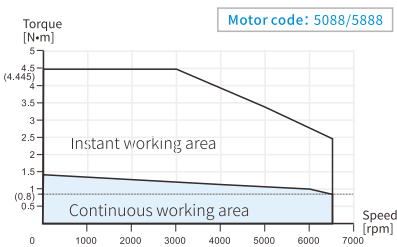
MS6H-60CM30B(Z)4-20P4
