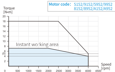
MS6G-130CM/CN/TL/TH20B(Z)2-41P5
