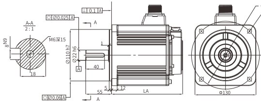
130 flange
