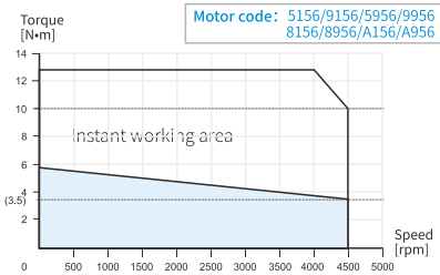
MS6G-130CM/CN/TL/TH15B(Z)2-41P5
