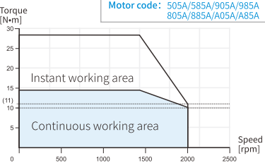
MS6G-180CN/TH15B(Z)2-44P4
