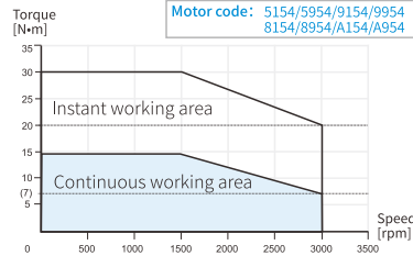
MS6G-130CM/CN/TL/TH15B(Z)2-42P3
