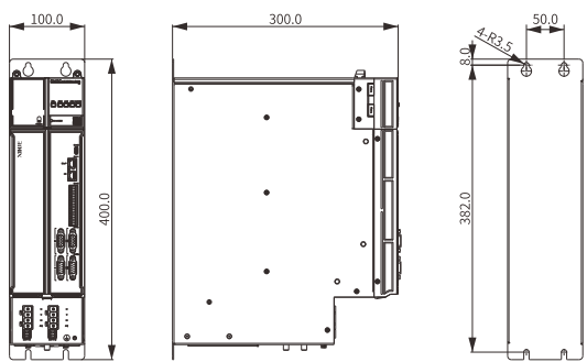
DM6C-45P5/47P5/415P0-M
