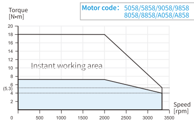
MS6G-130CM/CN/TL/TH20B(Z)2-21P5
