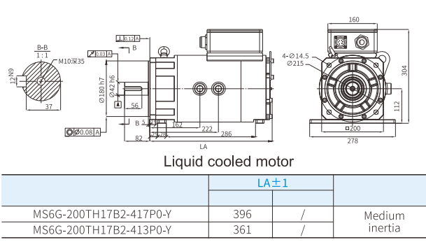
200 flange
