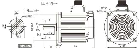
110 flange
