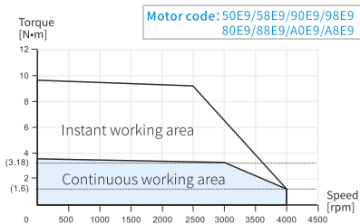
MS6H-80CM/CN/TH/TL30B(Z)3-21P0
