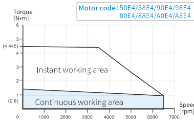
MS6H-60CM/CN/TH/TL30B(Z)3-20P4
