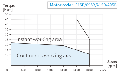
MS6G-180CN/TH15B(Z)2-43P0
