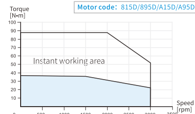
MS6G-180CN/TH15B(Z)2-45P5
