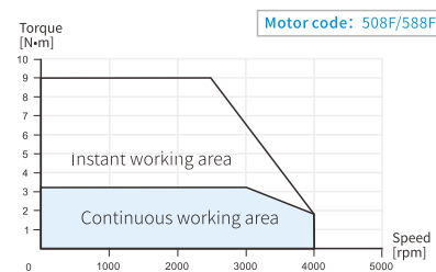
MS6H-80CM30B(Z)4-21P0
