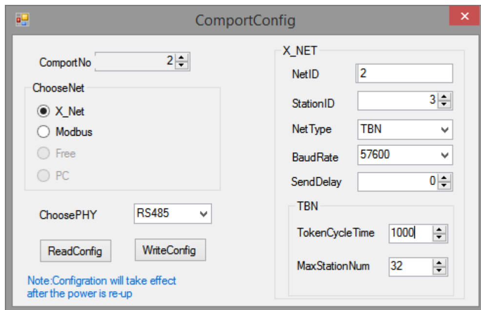
Fig. 3-2 TBN mode
