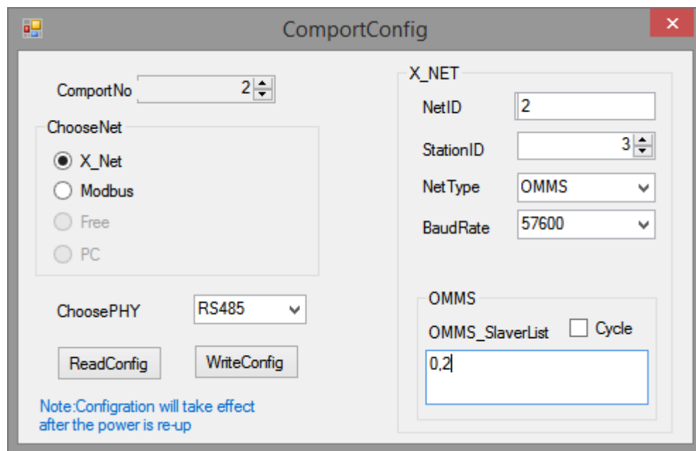
Fig. 3-1 OMMS mode
